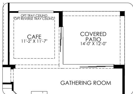
70495 - Open Corner Sliding Glass Door
