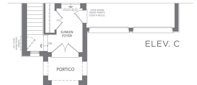
ELEV. B
