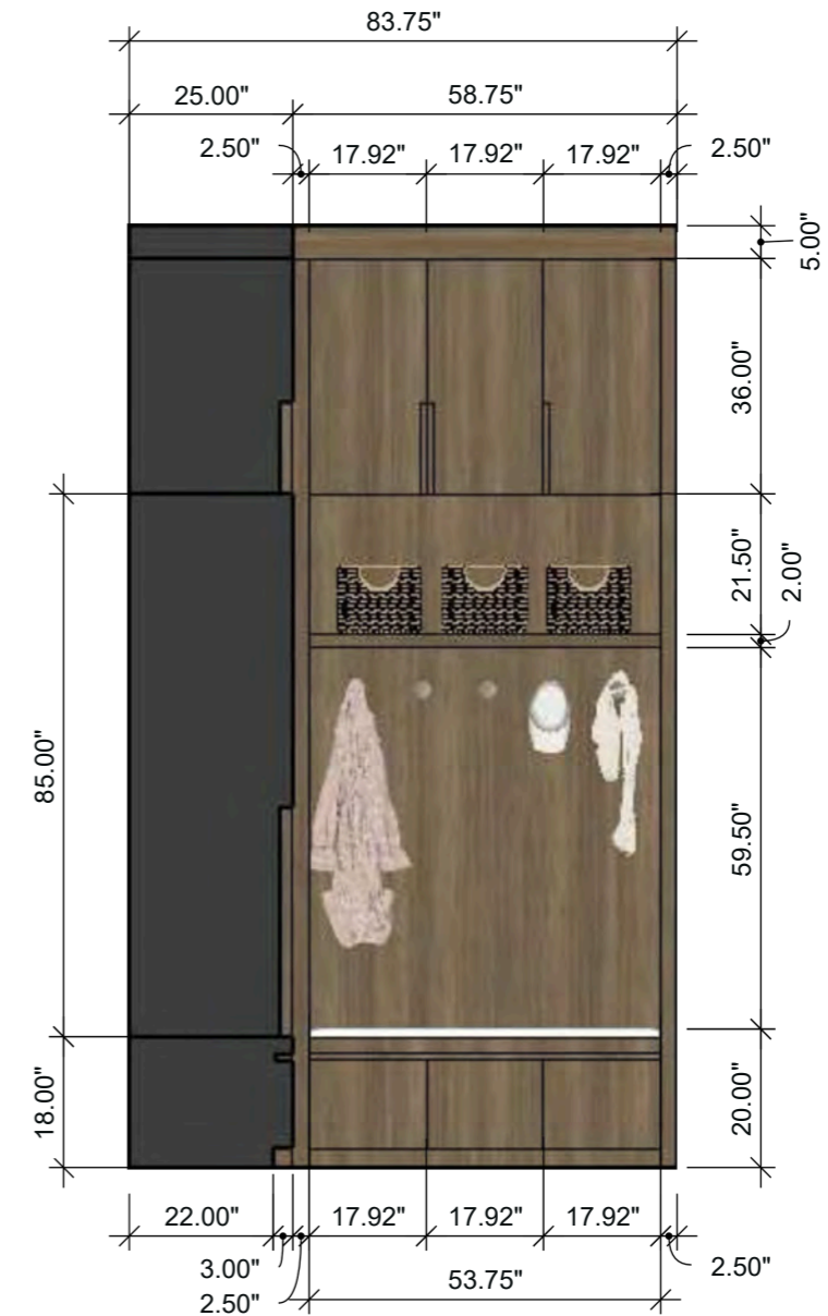
Mudroom Elevation 2 SCALE: 3/8" = 1'-0" (1:32)
