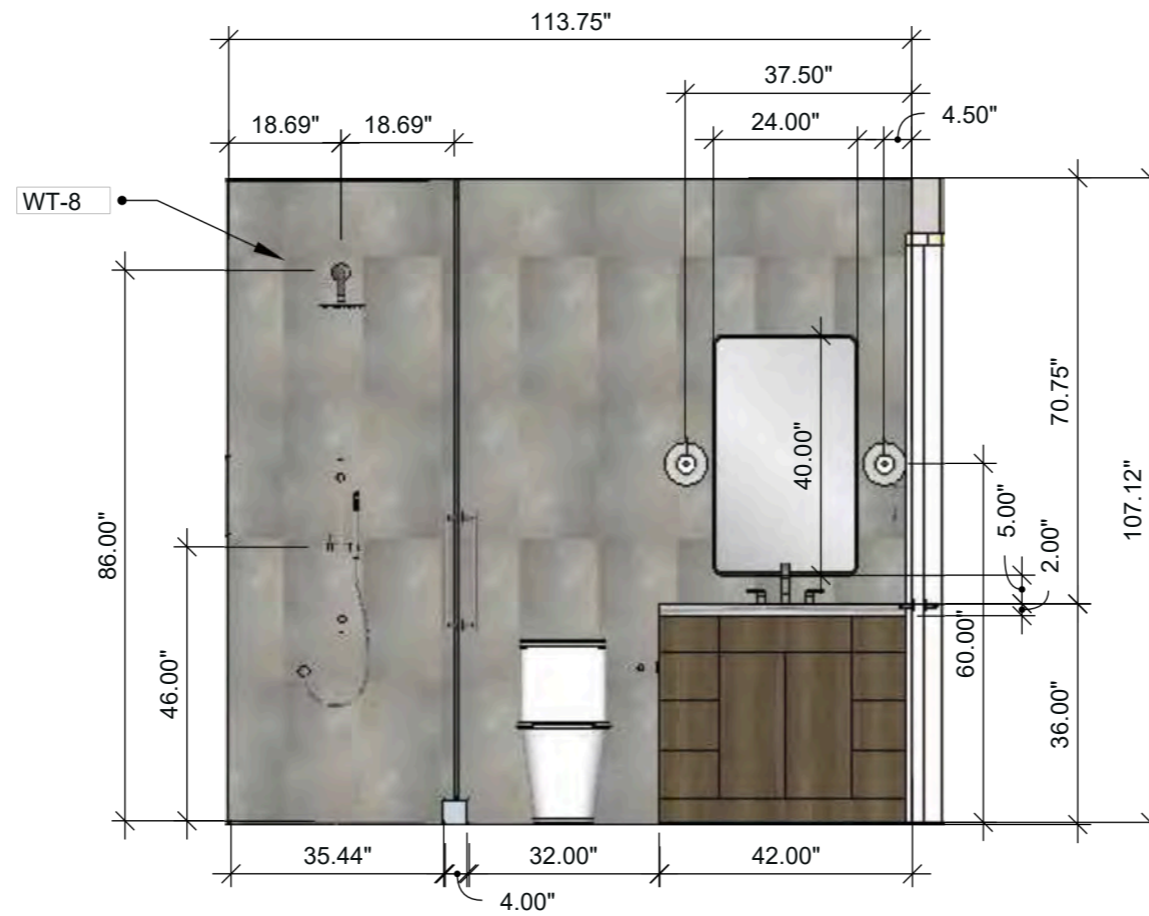
Bath 3 Elevation 1 SCALE: 3/8" = 1'-0" (1:32)
