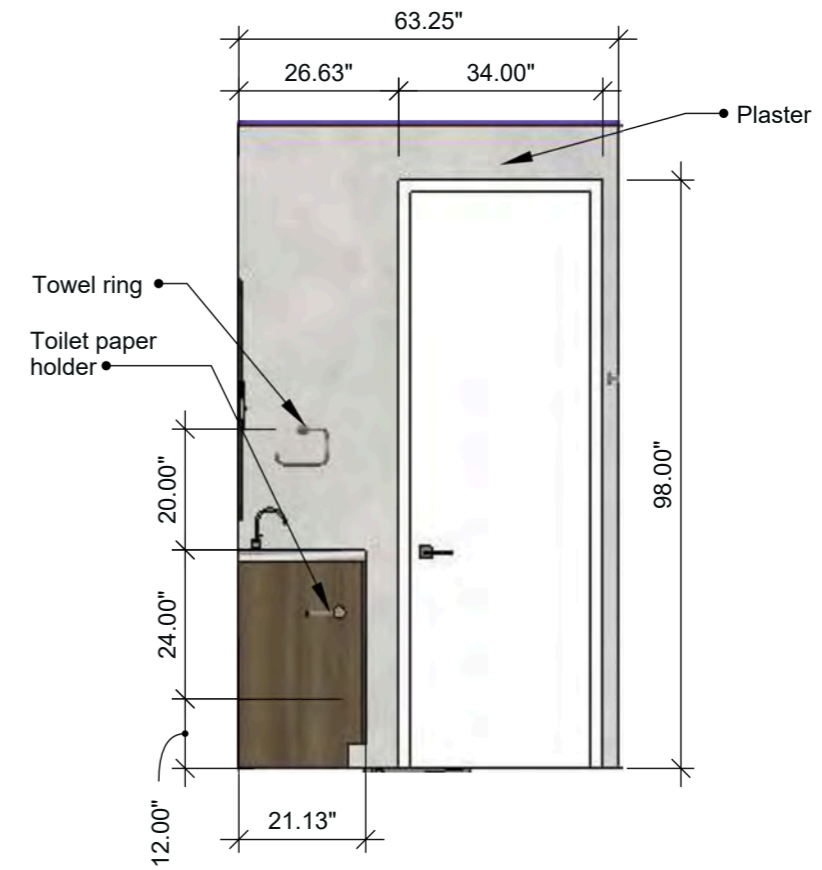
Bath 3 Elevation 2 SCALE: 3/8" = 1'-0" (1:32)
